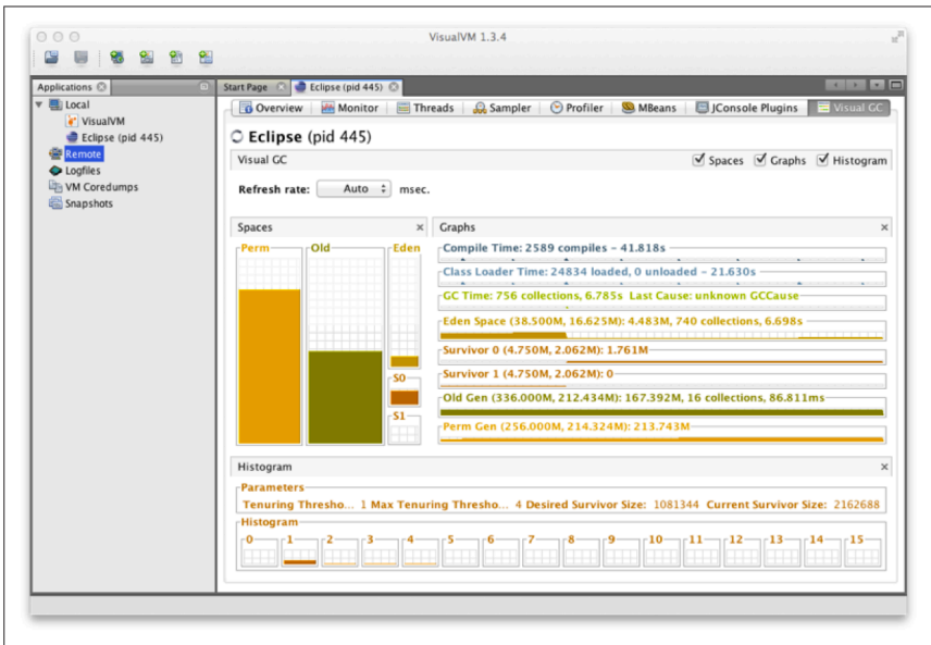
Figure A-7. VisualGC plug-in
