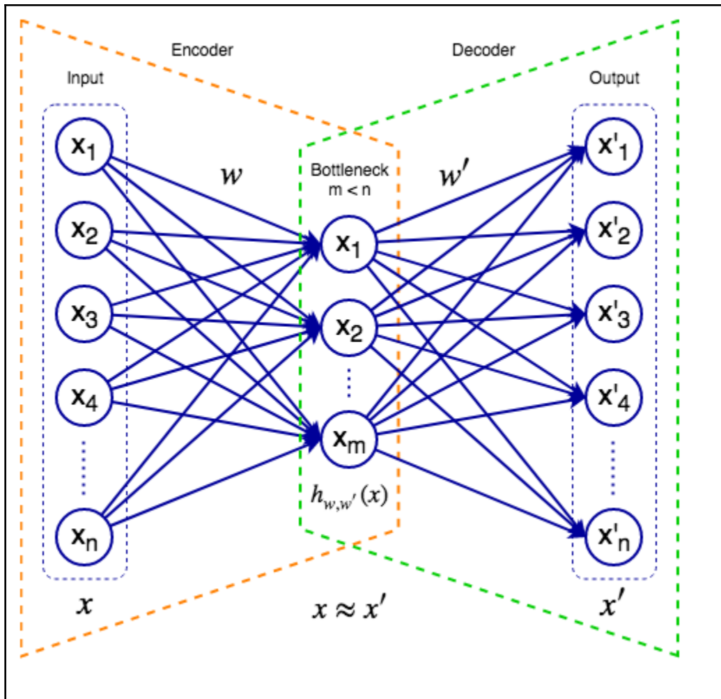
An autoencoder
